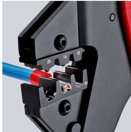
97 43 200 s lisovacím nástavcem 97 49 09 pro koncové dutinky kabelů
