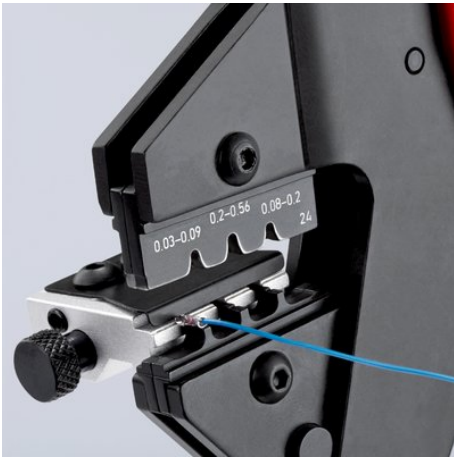
97 43 200 s lisovacím nástavcem 97 49 24 a polohovací pomůcka 97 49 93 pro konektory D-Sub
