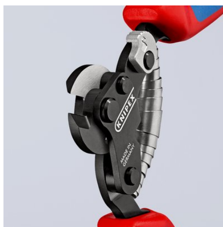
Dvojitě uložený kloub
