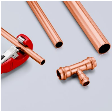
Para cortar tubos de cobre, latón y acero inoxidable y conductos rígidos de acero con espesor de hasta 2 mm y diámetros de 6 a 35 mm (1/4" - 1 3/8")
