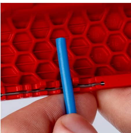
90 22 02 SB: Ingiuten längdskala för jämn avisolering av kablarna till enhetlig längd, läsbar för höger- och vänsterhända
