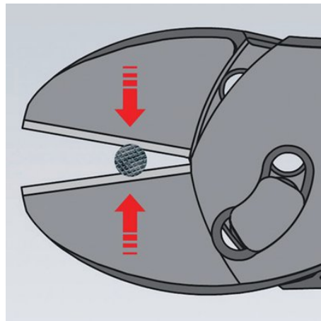
Vajrarna läggs alltid in så nära leden som möjligt. På högutväxlade klippverktyg är öppningen nära vridpunkten för det mesta mindre än vajerns tjocklek och vajrarna kan glida framåt vid klippning.
