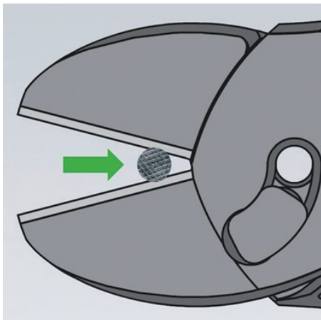
Gör först en skära i vajern med KNIPEX TwinForce® till nödvändig handkraft ökar avsevärt. Öppna nu tången och skjut in vajern i skåran längre in mot leden.
