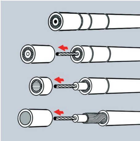
Driedelig afstrippen van een coax-kabel
