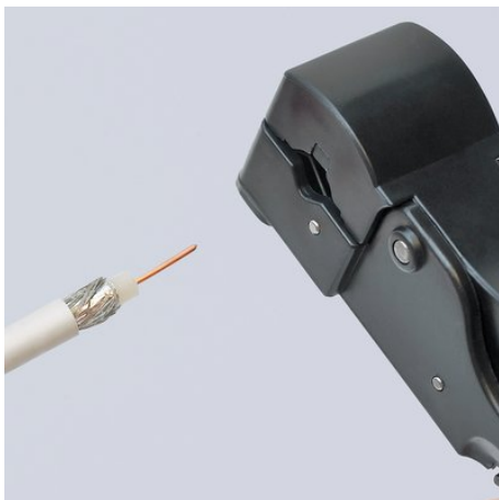
Binnenlagen een voor een vrijgelegd
