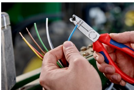
Avisoleringshål för ledarareor 1,5 och 2,5 mm 2
