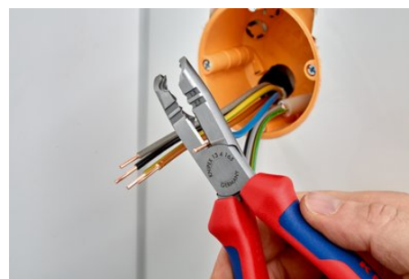
Knippen bij inkorten van individuele geleiders
