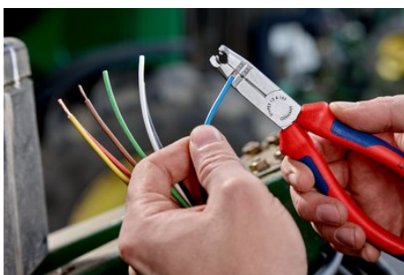
Isolatiegaten voor geleiders 1,5 en 2,5 mm 2
