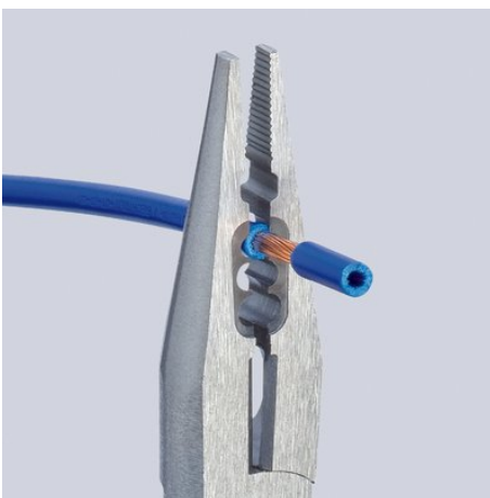
Stripping 0,5 - 0,75 / 1,5 / 2,5 m 2
