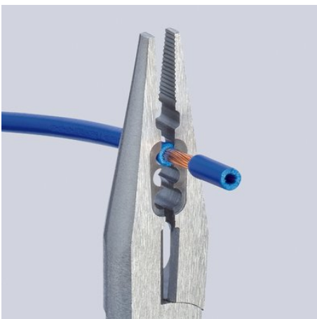
Odizolování 0,5 - 0,75 / 1,5 / 2,5 mm 2
