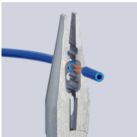
Odizolování 0,5 - 0,75 / 1,5 / 2,5 mm 2
