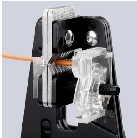
Perfekt inskärning av isolationen längs hela periferin
